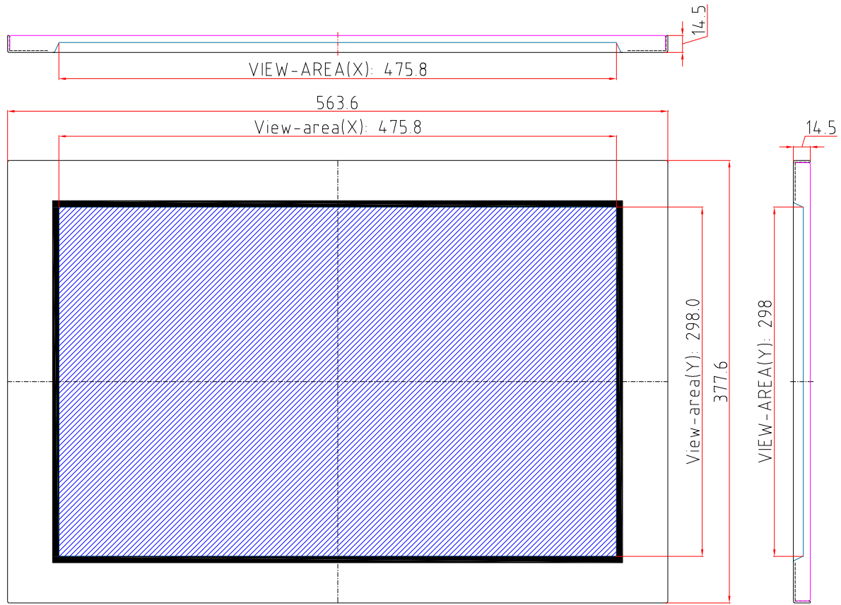
(22"IR-TOUCH : FRONT-VIEW)
